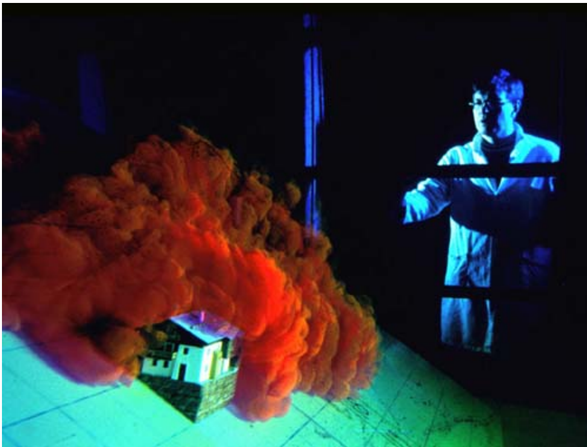
Essai en laboratoire (Cemagref) visant à reproduire une avalanche en aérosol.
